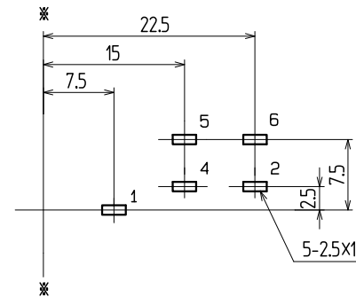
て1.6 参考基板孔寸法 (パターン面) (公差 ALL ±0.1) (数字は端子番号を示す)
