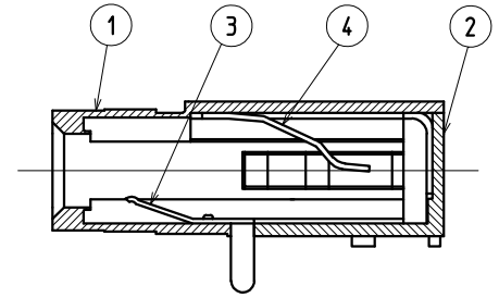
A-A 断面図
