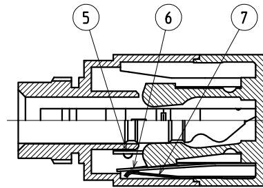
B-B 断面図
